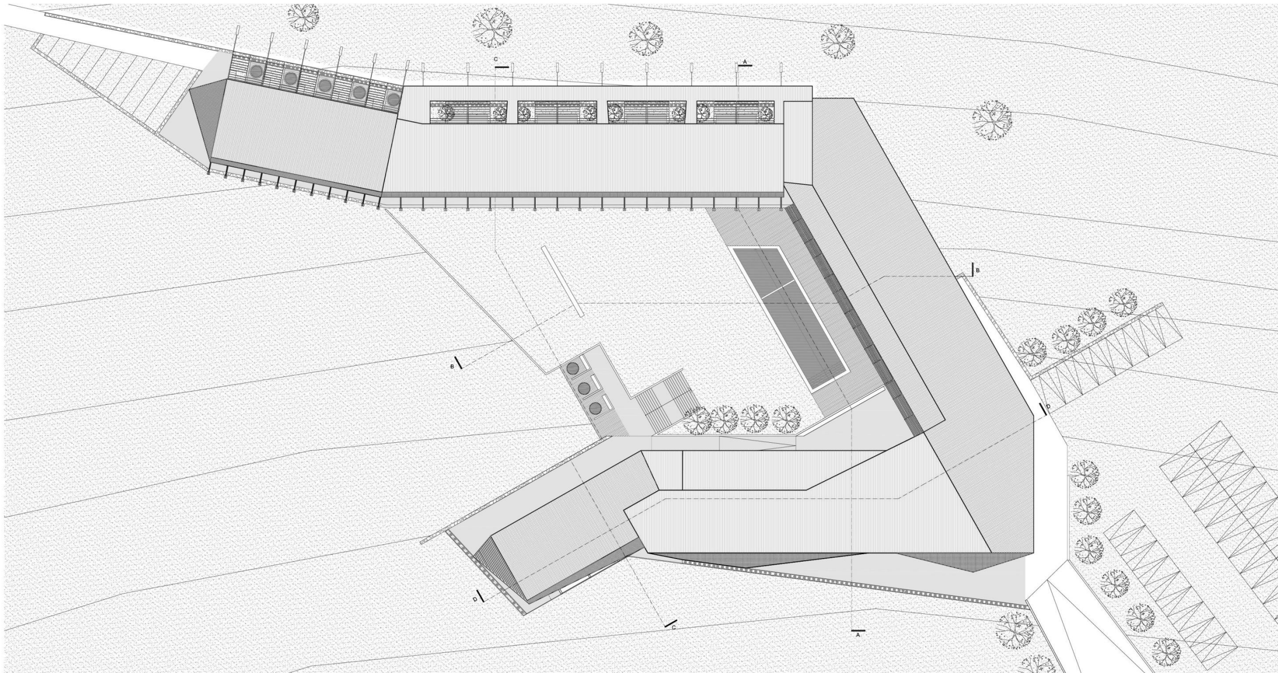
PLANTA CUBIERTA
