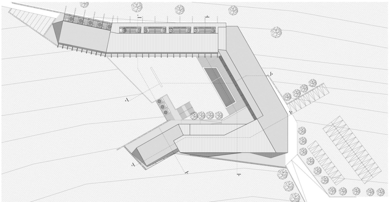
PLANTA EMPLAZAMIENTO
