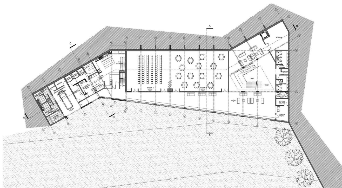
PLANTA SUBTERRANEO
