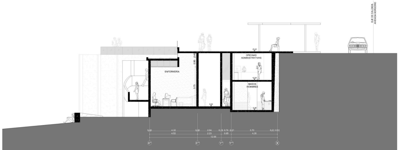
CORTE B-B'
