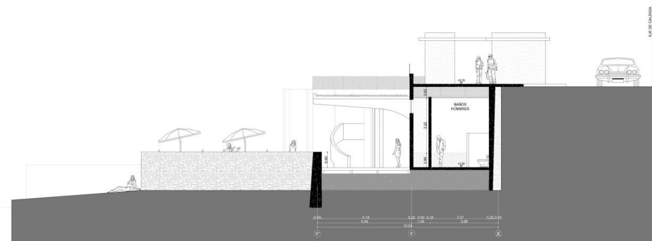
CORTE A-A'
