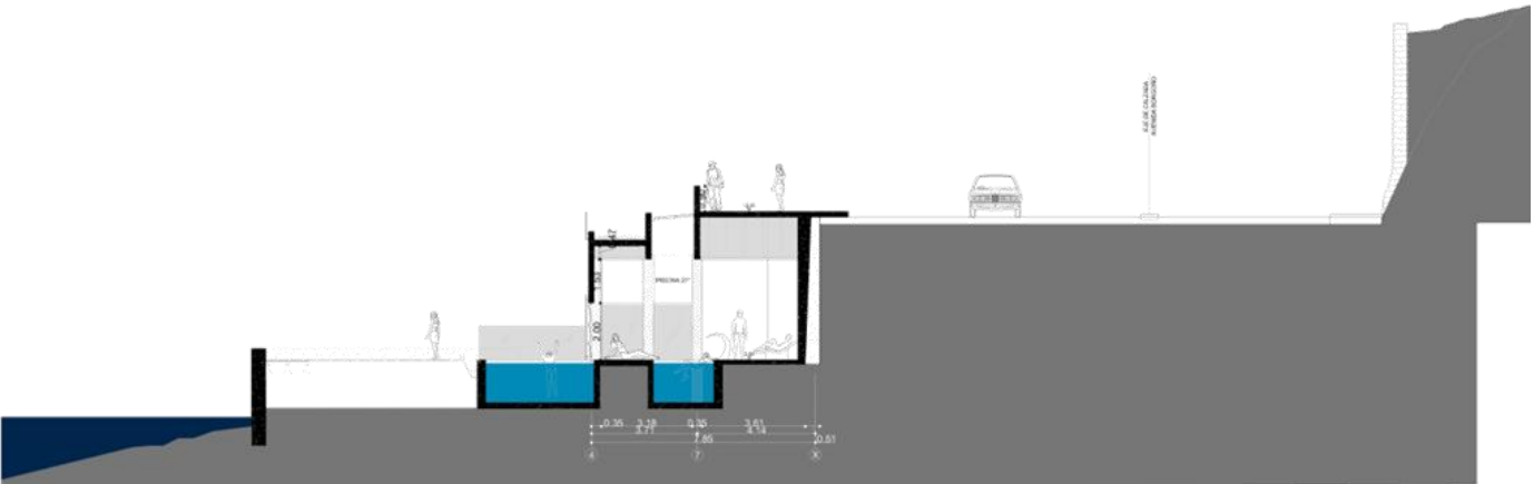
SECCION E-E'
