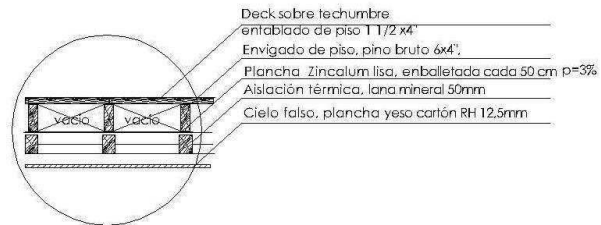
Longitudinal
