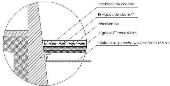
Transversal
